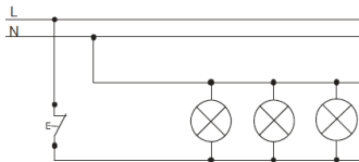
Abbildung: Notstromkreis
